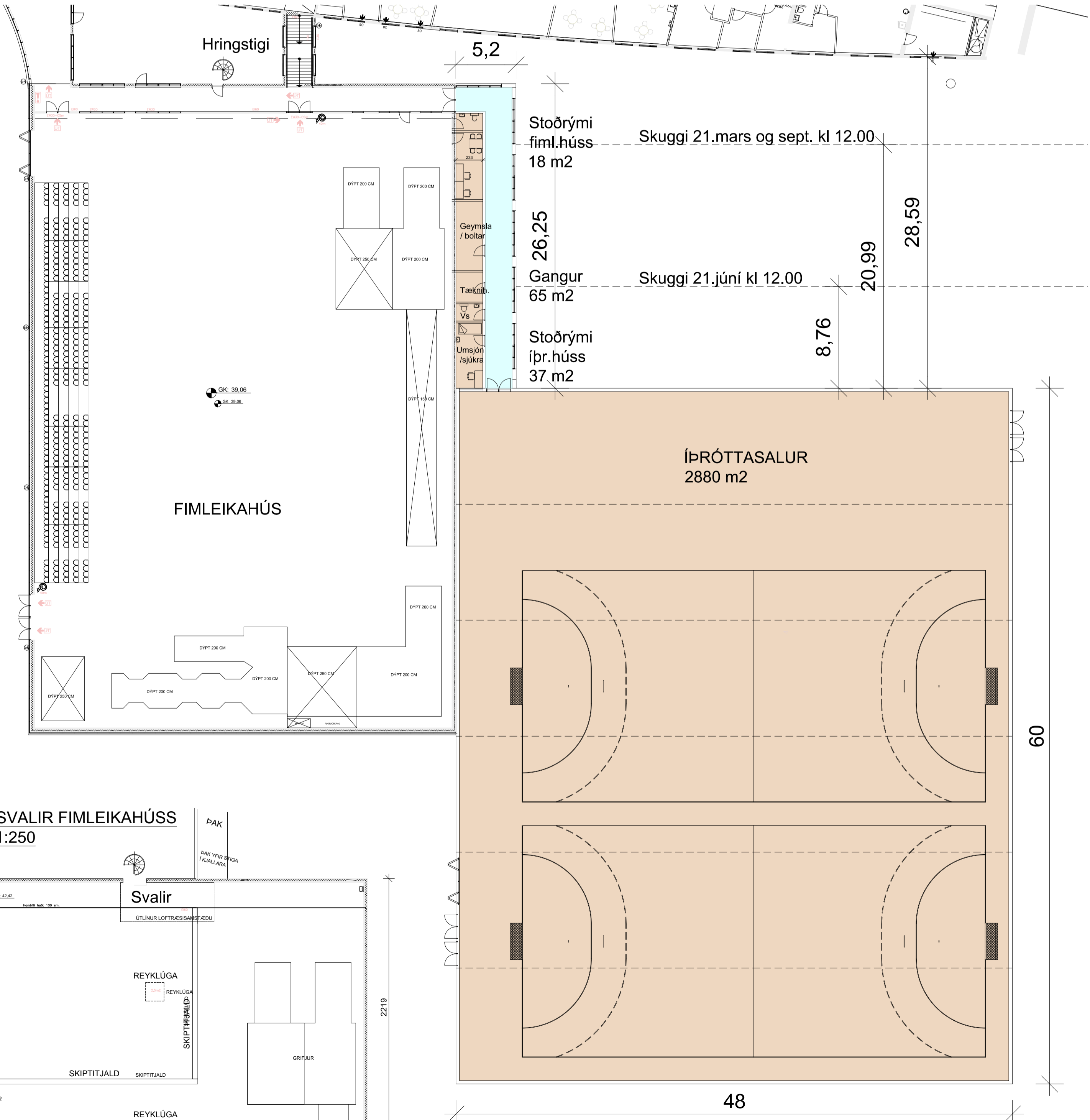
GRUNNMYND 2880 m 2 +140 m 2 = 3020 m 2 1:250
